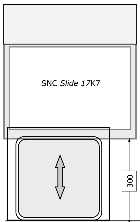
Vue de Dessus: Tiroir ouvert
