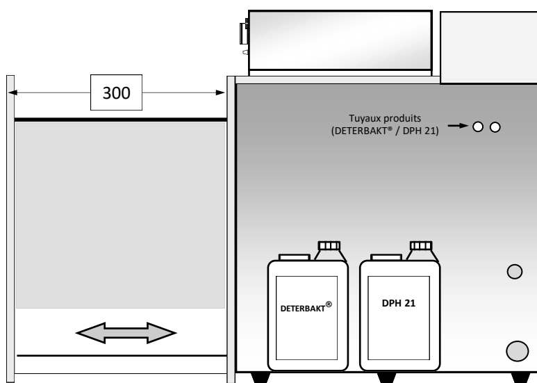
Vue de Côté : Tiroir ouvert
